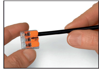
Lower the lever to close the clamp Baje la palanca para cerrar la abrazadera
