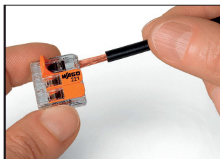
Lift the lever to open the clamping unit and insert a stripped conductor. Levante la palanca para abrir la unidad de sujeción e inserte un conductor pelado.
